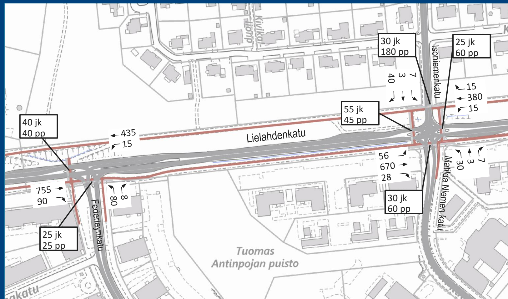
Kuva: Simulaatiossa käytetyt ennustevuoden 2040 iltahuipputunnin (IHT) liikennemäärät
