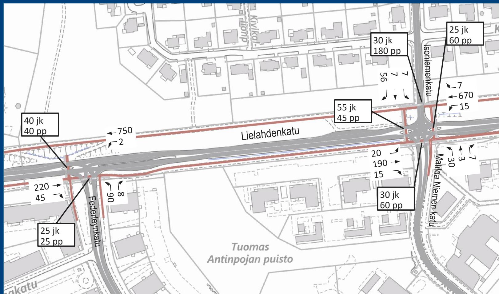
Kuva: Simulaatiossa käytetyt ennustevuoden 2040 aamuhuipputunnin (AHT) liikennemäärät
