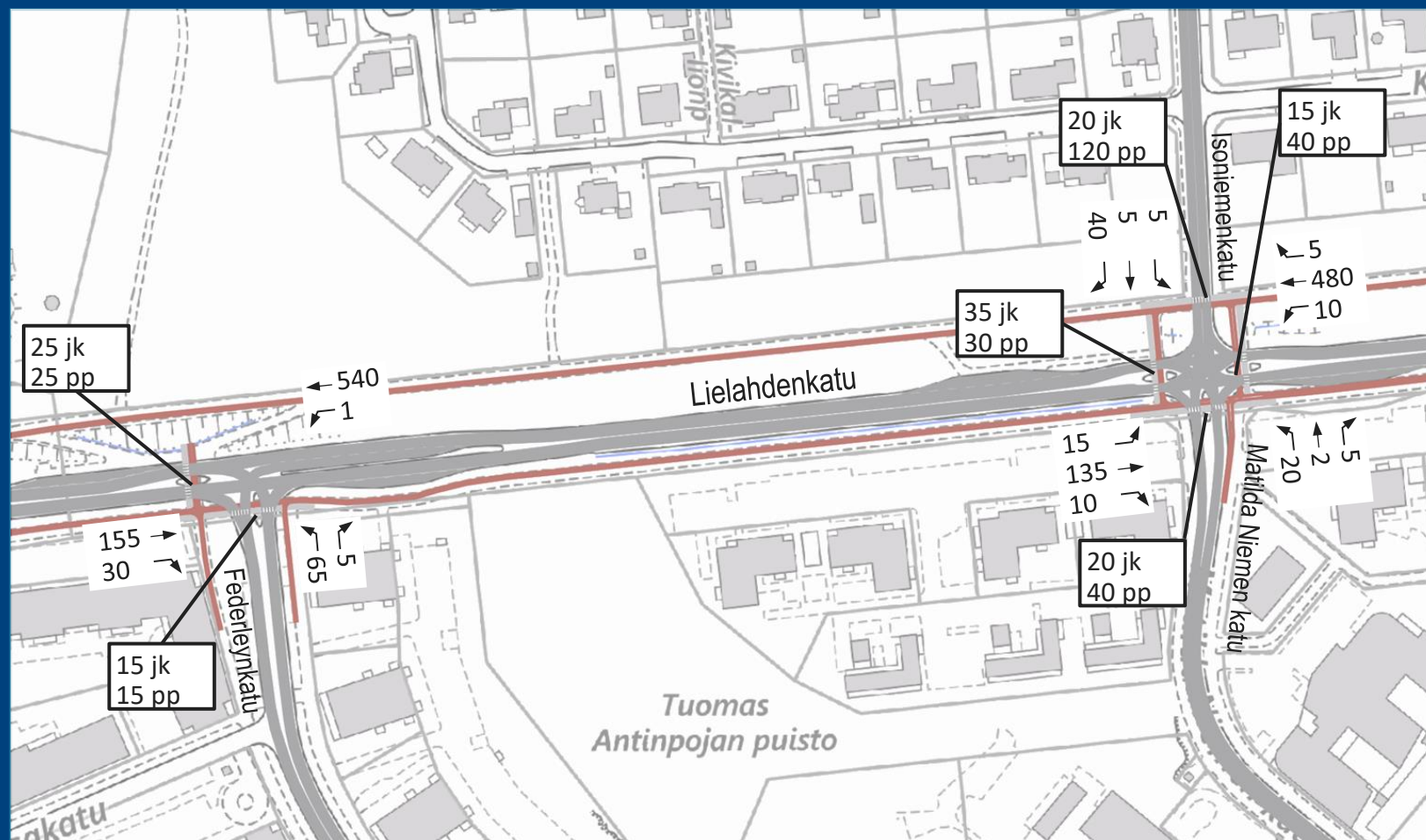
Kuva: Simulaatiossa käytetyt liikennemäärät nykytilan aamuhuipputuntina (AHT)
